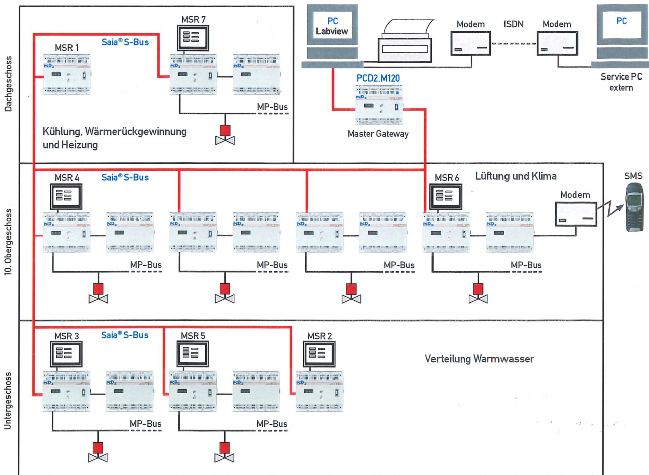
GA-Kommunikationsschema Accor-Hotel Bern Expo
