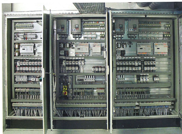
Schaltschränke mit den Unterstationen Saia®PCD2.M120 plus Erweiterungsgehäusen
